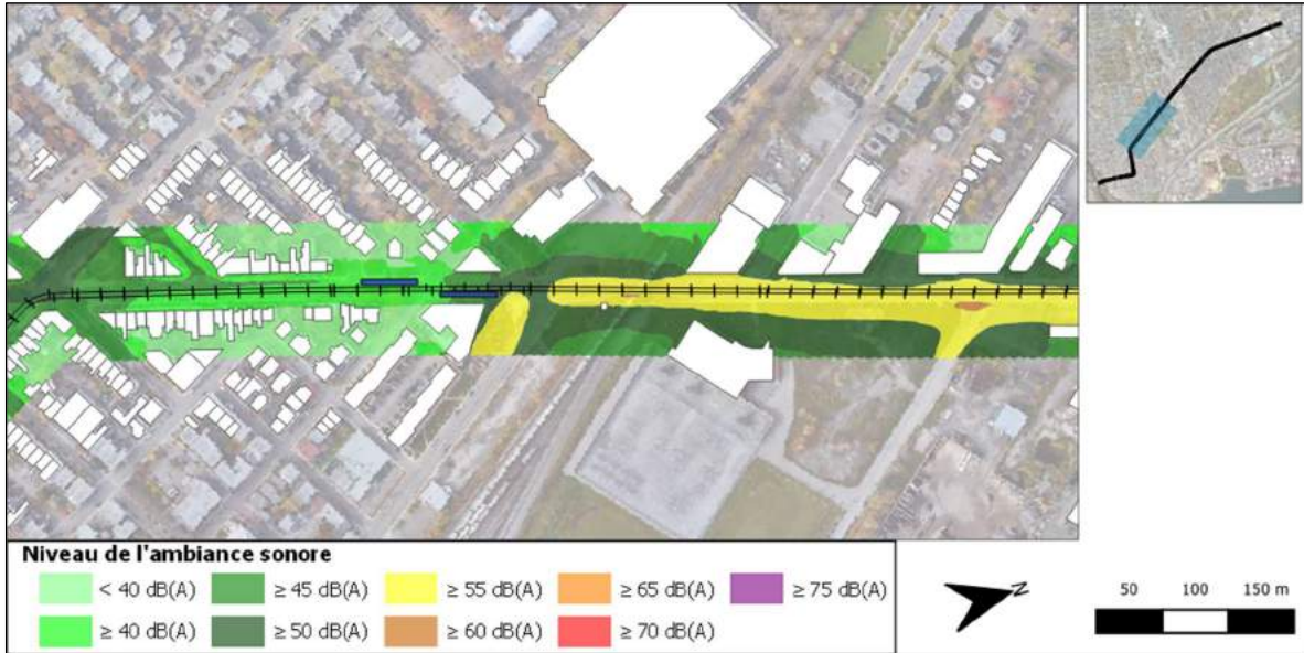
Figure 41 : Cartographie des niveaux de bruit ambiant en 2026 dus à la circulation routière Secteur du chemin de la Canardière, entre l'intersection de la 4 e Avenue et le boulevard Henri-Bourrassa Niveau de bruit en période nocturne L_n – Hauteur 4m
