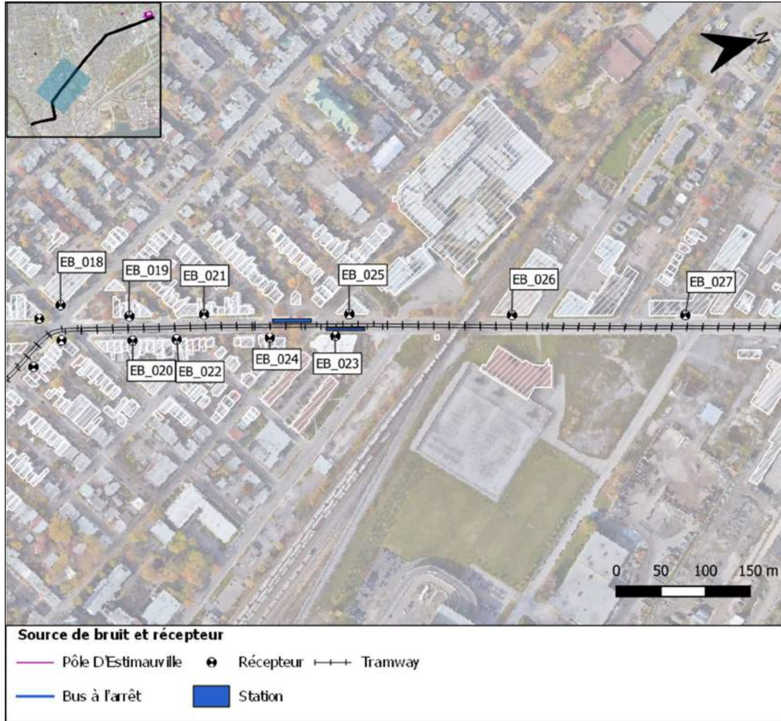
Figure 4 : Sélection des bâtiments représentatifs pour l'étude acoustique détaillée au niveau du chemin de la Canardière, entre l'intersection de la 4 e Avenue et le boulevard Henri-Bourassa
