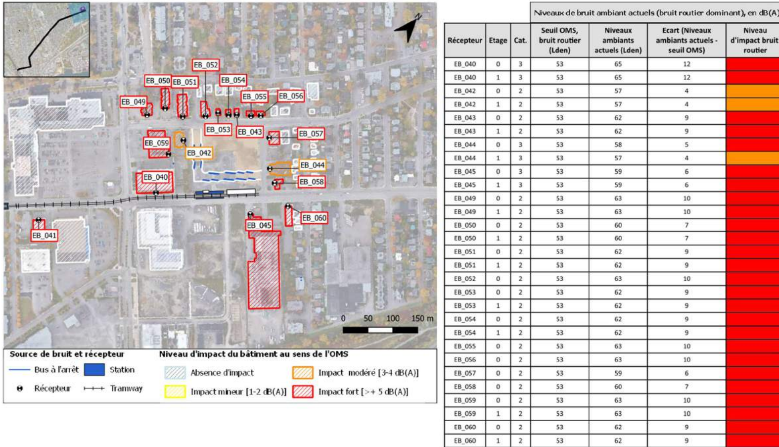
Figure 61 : Niveaux sonores et niveaux d'impact du bruit ambiant actuel (bruit routier dominant) par rapport aux recommandations de l'OMS – Secteur du Pôle D'Estimauville– Niveau de bruit L_{DEN}
